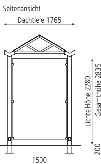
Wartehalle WAAGE, Dachbreite x Dachtiefe 6400 mm x 1765 mm, Rück- / Seitenwände ESG, Klarglas, mit Siebdruckdekor Raute, Drahtgittersitz TARVIS, Stahlkonstruktion in RAL 6024 verkehrsgrün
