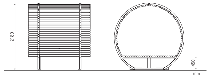
▲ Freizeitüberdachung CISON CONTEA mit Liegefläche, kreisförmig, mit Kiefernholzbelattung, Stahlteile in RAL 7016 anthrazitgrau
