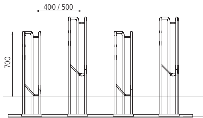
▲ Radeinstellung einseitig tief/hoch zum Aufdübeln bei -200 mm
