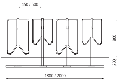
▲ Radeinstellung doppelseitig hoch/tief, zum Aufdübeln bei -200 mm (Reihenaufstellung)
