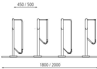
▲ Radeinstellung einseitig tief/hoch, zum Aufdübeln (Reihenaufstellung)
