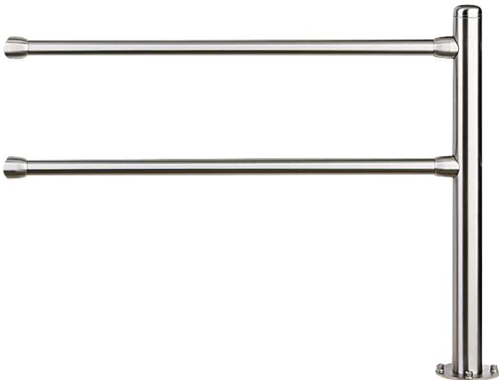
Ergänzungsset Geländersystem BORVO ohne Handlauf, mit Rundkopf, 1 m, zum Aufdübeln
