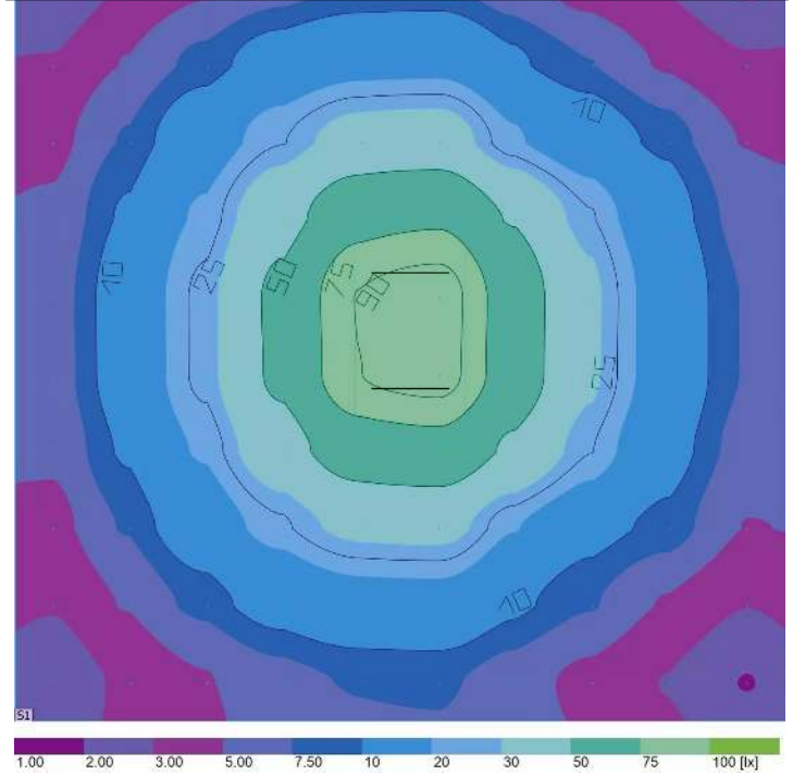
Beleuchtungsschema für 2 Felder
