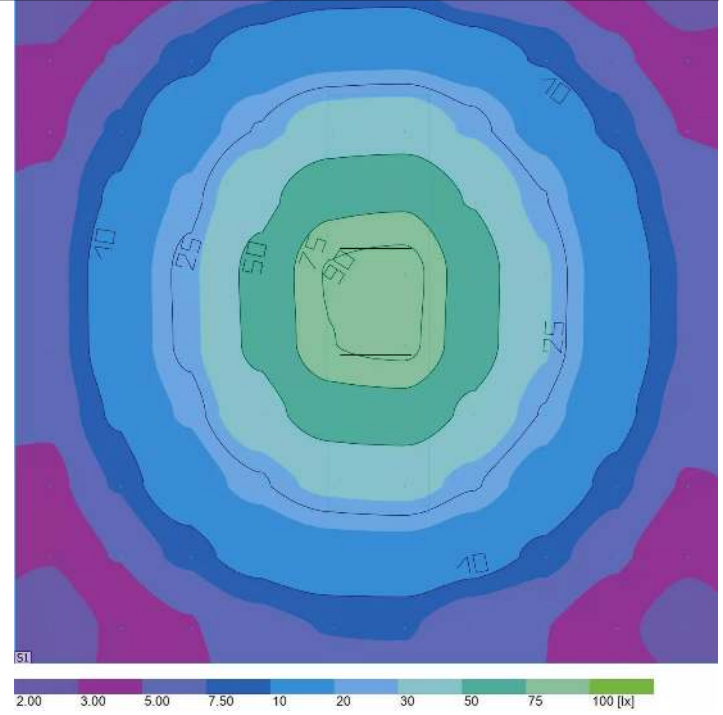
Beleuchtungsschema für 4 Felder
