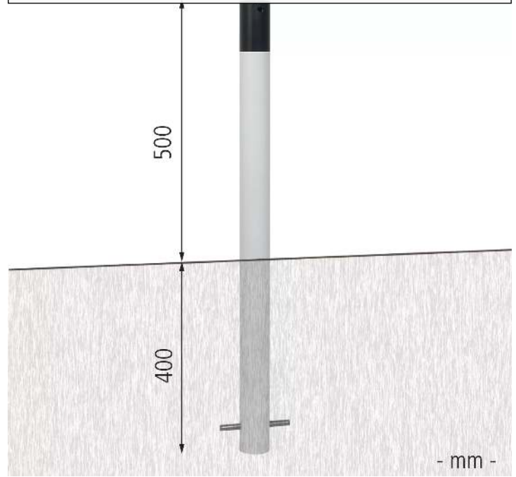
Feuerwehrleitpfosten TURKU
