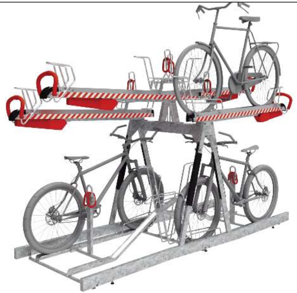
Doppelstock-Fahrradparksystem EASYLIFT 500 D, doppelseitig, 8 Stellplätze
