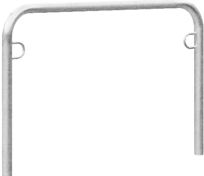
Anlehnbügel MIAMI NEW zum Einbetonieren, Breite 1500 mm
