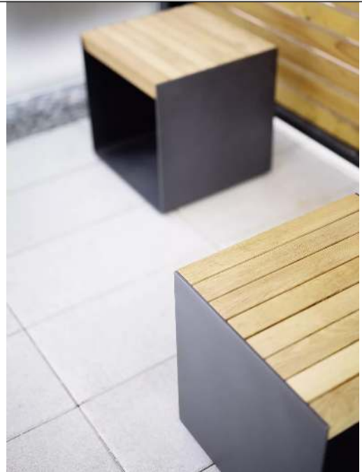
Sitz RADIUM mit Robinienholzbelattung, Stahlteile in RAL 7016 anthrazitgrau
