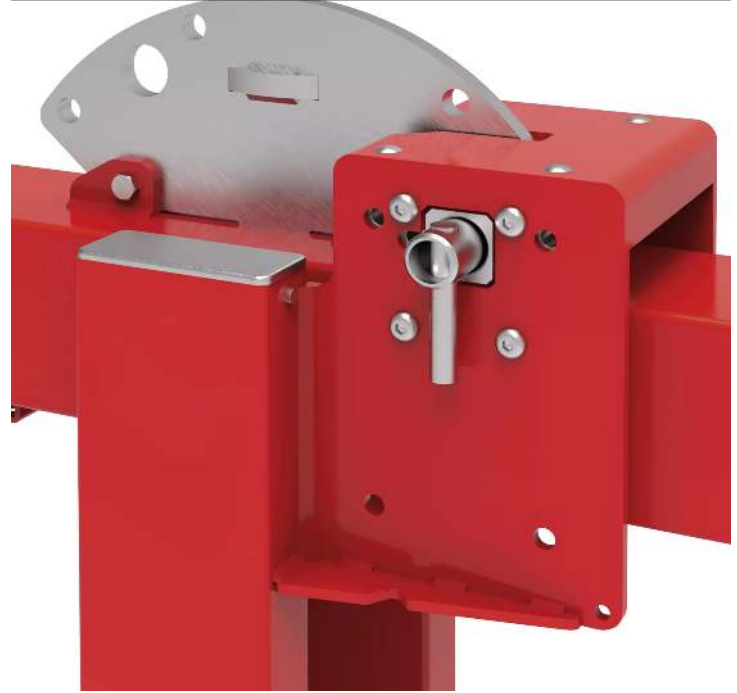
Standardverriegelung durch Bolzen für Vorhängeschloss
