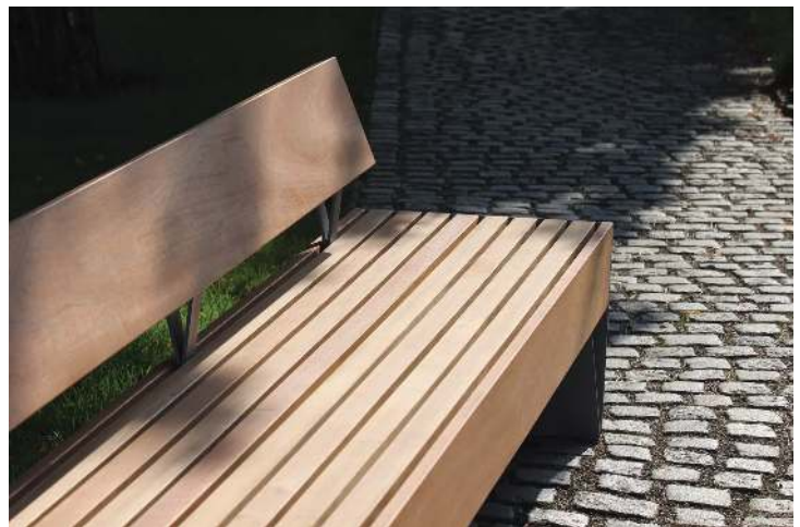
Sitzbank BLOCQ mit Rückenlehne, mit Jatobaholzbelattung, Stahlteile in RAL 9007 graualuminium
