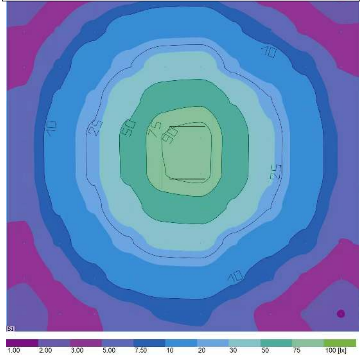
Beleuchtungsschema für 2 Felder
